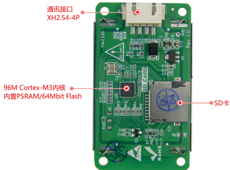
图 1-2 硬件配置图
