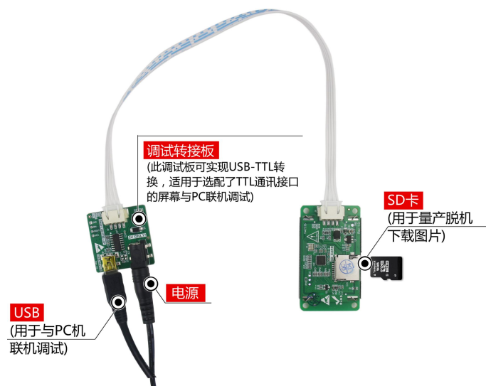
图 1-3 调试工具图
