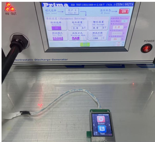
图 5-2 ESD 测试图
