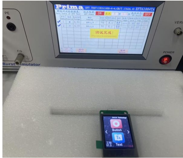
图 5-4 群脉冲测试图
